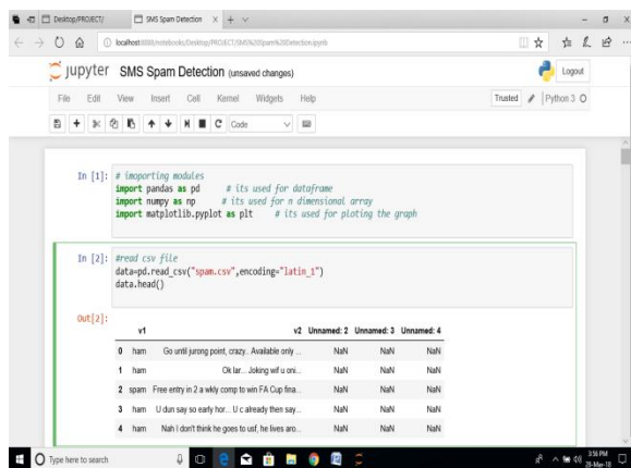
Fig.4.1. DATA set.
